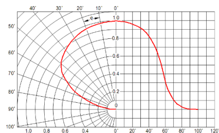
Рисунок 3 Типы КСС
