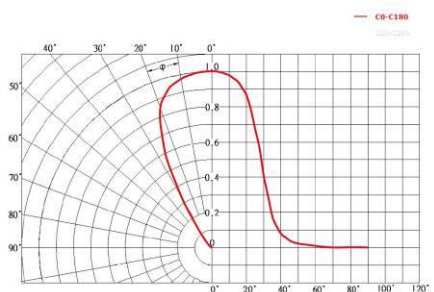
Рисунок 3 Типы КСС
