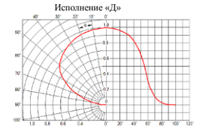
Рисунок 3 Тип КСС
