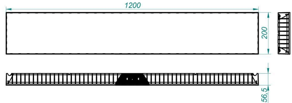
Рисунок 16 Светильник L-school 32
