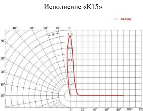
Рисунок 8 Тип КСС
