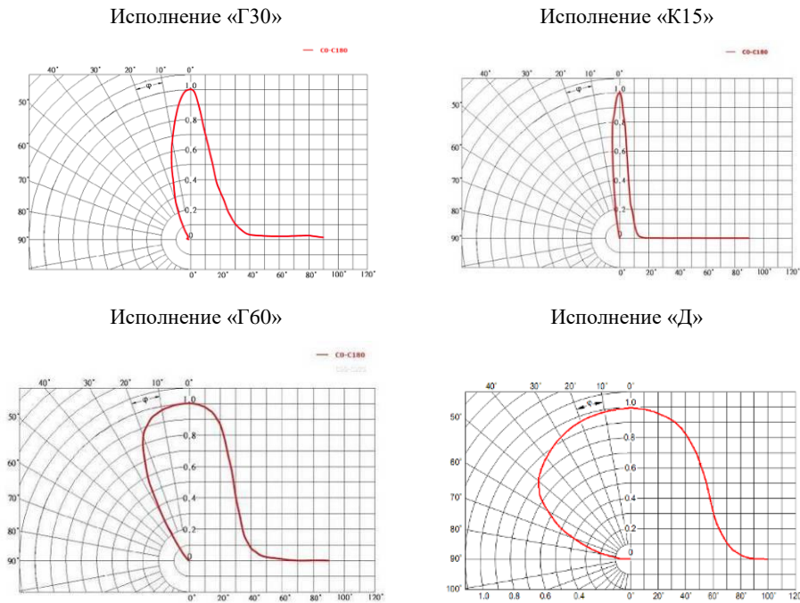
Рисунок 4 Типы КСС
