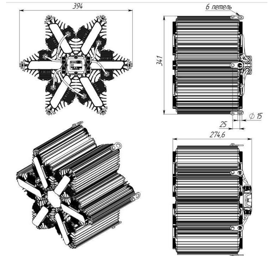
Рисунок 1 Светильник «L-lego 330». Подвесное крепление
