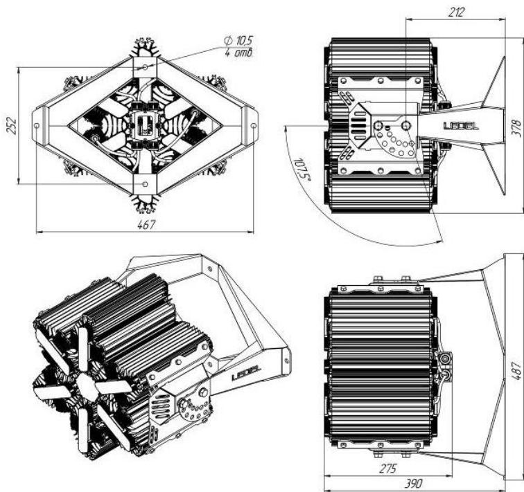
Рисунок 2 Светильник «L-lego 330 banner» Поворотное крепление
