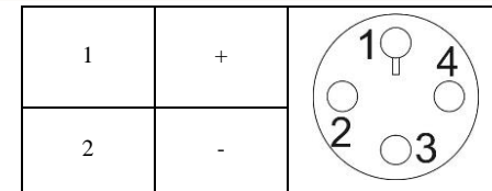
Рисунок 4 Схема подключения модуля
