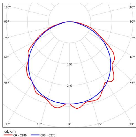
Рисунок 4 Типы КСС
