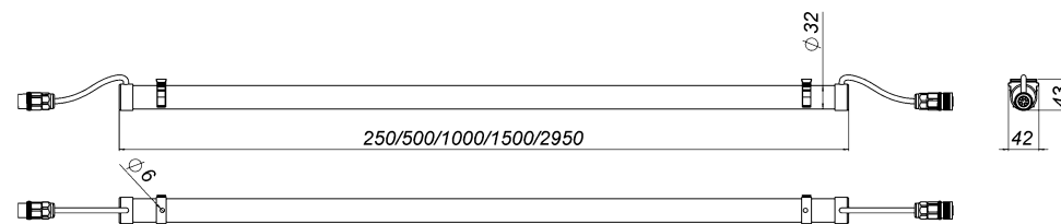
Рисунок 2 Модуль «L-line».
