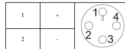
Рисунок 4 Схема подключения модуля
