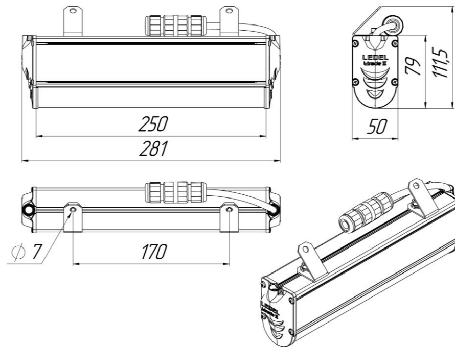
Рисунок 1 Светильник «L-trade II 12 с фиксированным угловым креплением»
