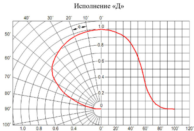
Рисунок 5 Тип КСС
