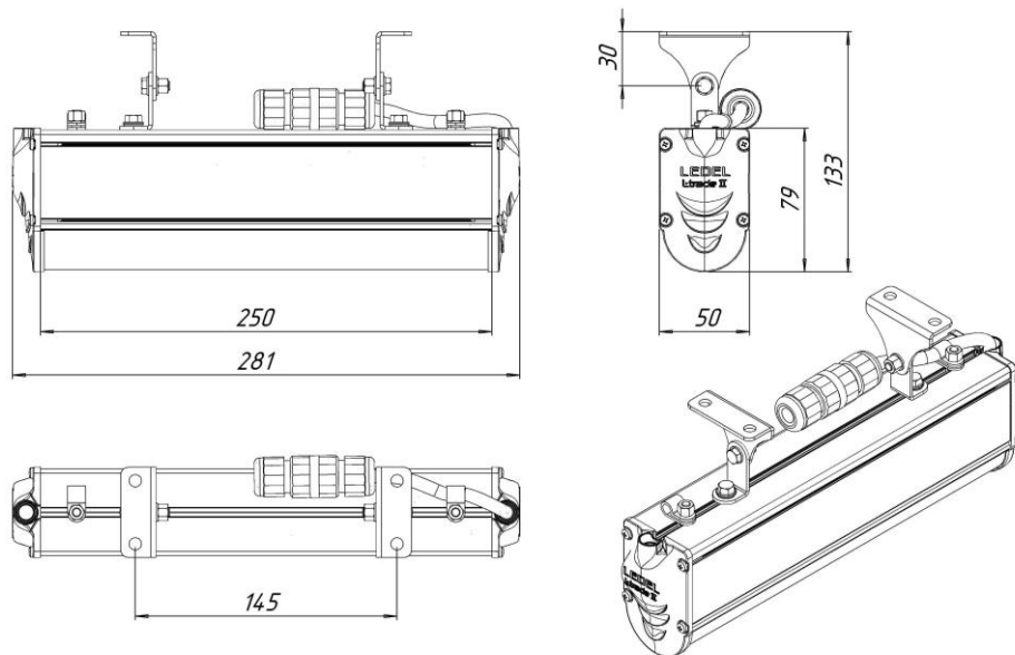
Рисунок 2 Светильник «L-trade II 12 с поворотным креплением»
