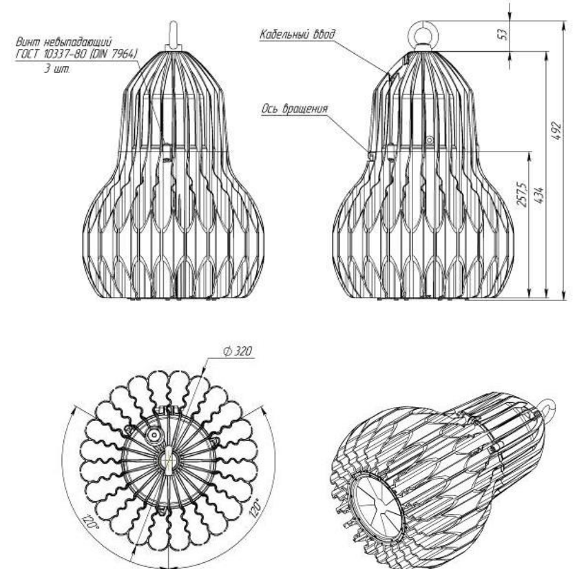
Рисунок 1 Светильник «L-industry 115/230»
