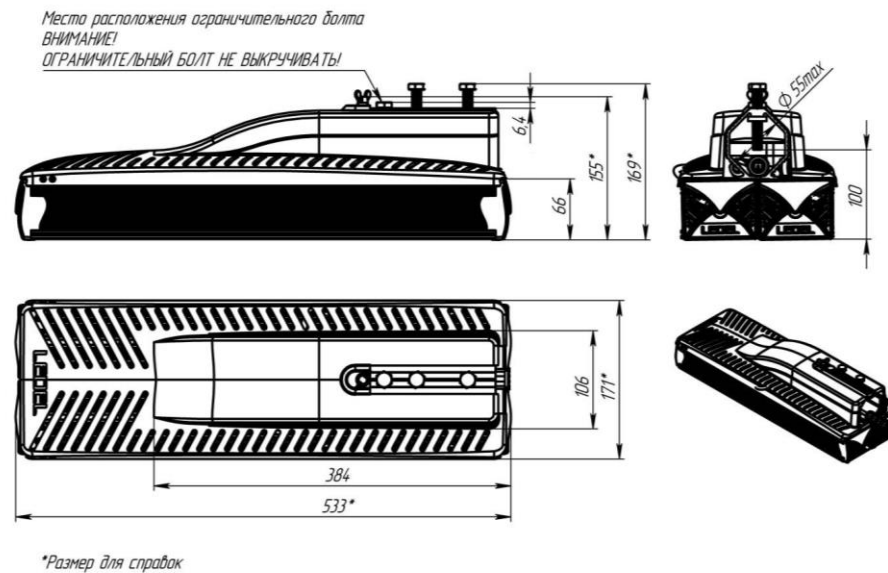
Рисунок 1 Габаритные размеры светильника «L-street 48»
