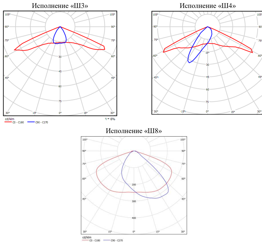
Рисунок 3 Типы КСС
